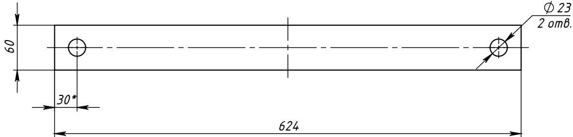
Поз.4 (Полухомут) развертка
